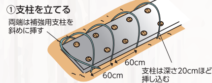
図 トンネルの作り方
