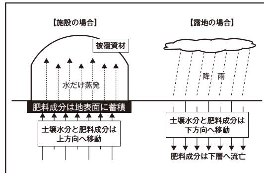
図20 施設土壌での水と肥料成分の動き
